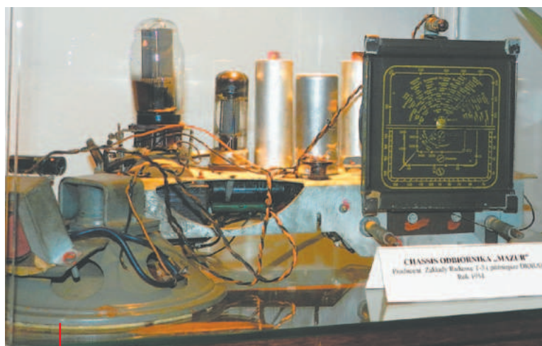
Chassis radioodbiornika Mazur (połowa lat 50. XX w.)
