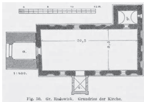
Fig. 50. Gr. Radowisk. Grundriss der Kirche.
